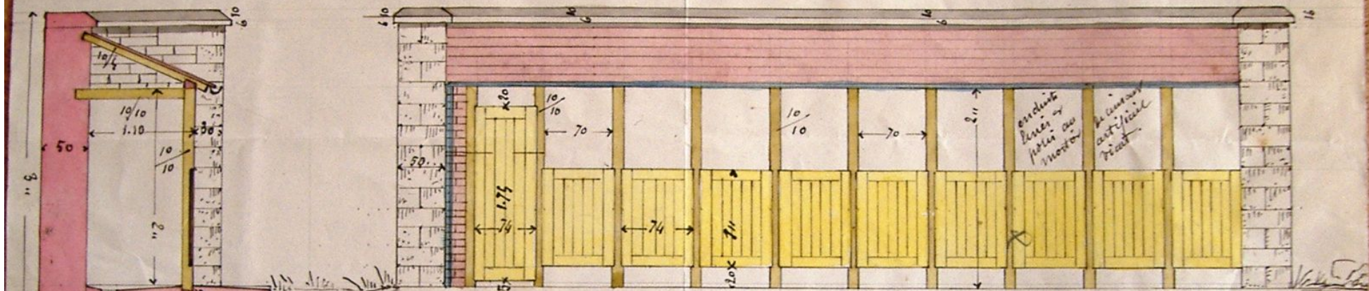
Elevation des cabinets
